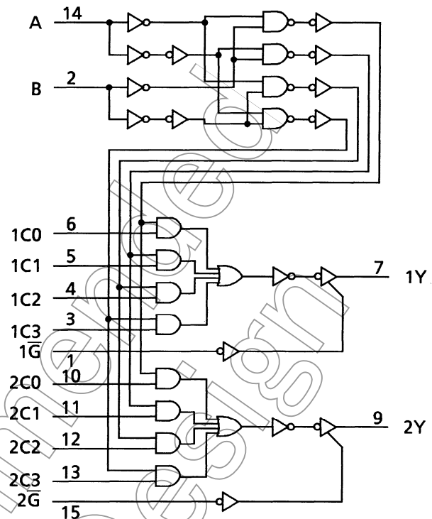
TC74HC253A
