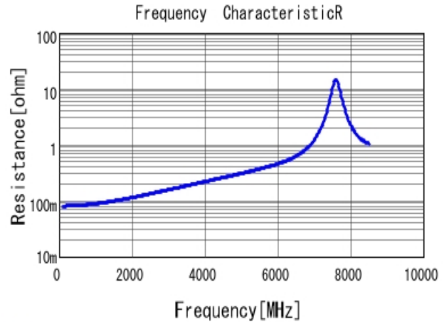
■ GCQ1555C1H8R8DB01 R DC0V, 25degC
