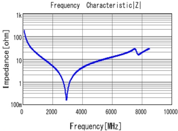
■ GCQ1555C1H8R8DB01 |Z| DC0V, 25degC
