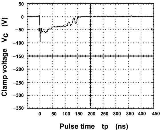
Fig. 11.2 -8 kV
