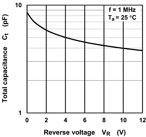
Fig. 9.3 C_t - V_R
