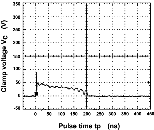
Fig. 11.1 +8 kV
