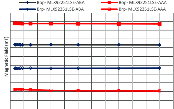
10.2. Magnetic parameters vs. V_{DD}
