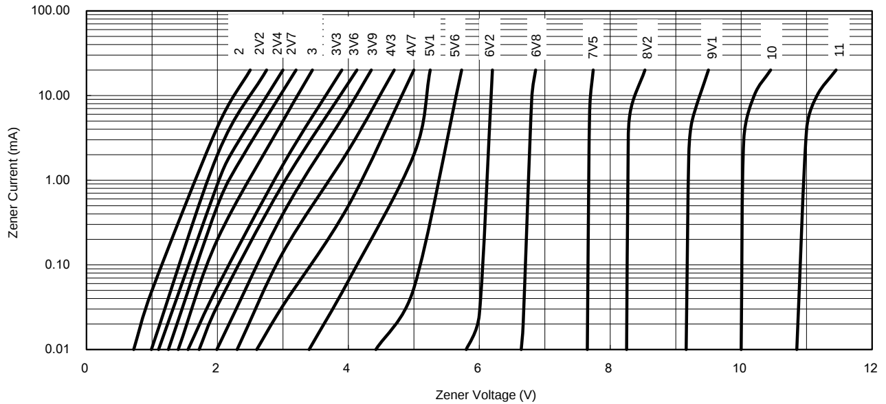
Fig. 7 Zener Voltage VS. Zener Current
