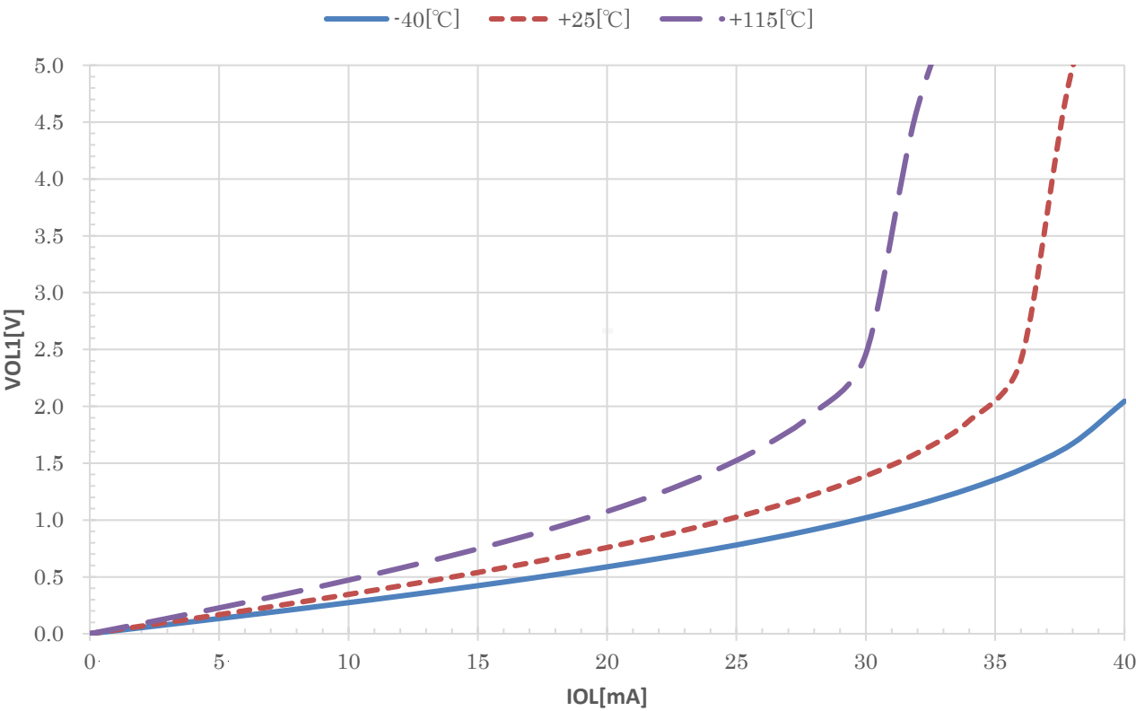
– VOL1 vs IOL (VDD=5V TYP.)
