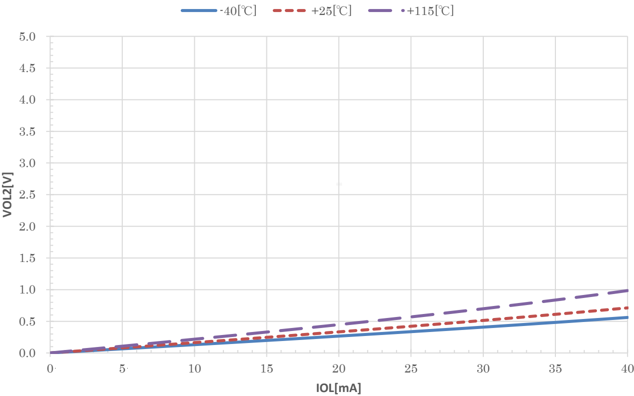
– VOL2 vs IOL (VDD=5V TYP.)
