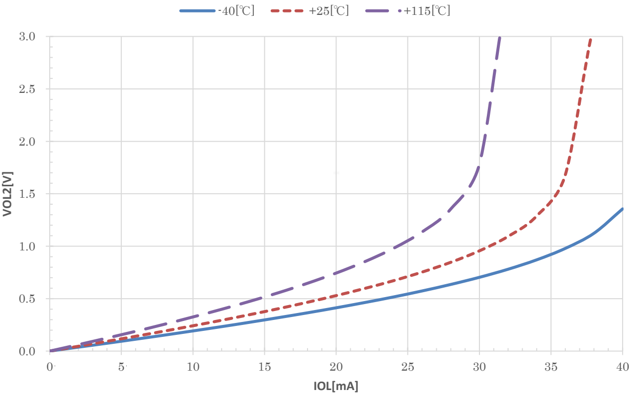
– VOL2 vs IOL (VDD=3V TYP.)
