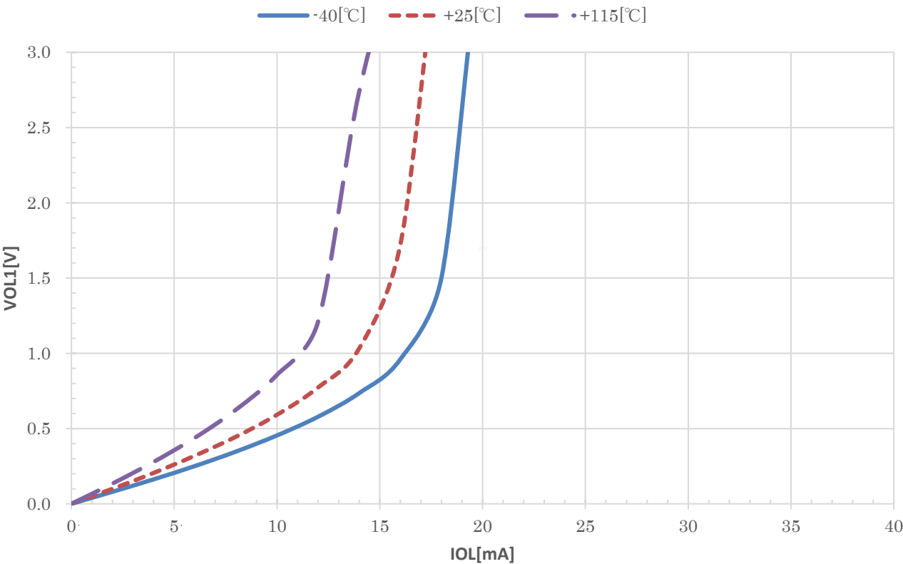
– VOL1 vs IOL (VDD=3V TYP.)
