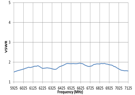
6 / 7 GHz VSWR
