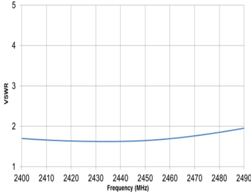
2.4 GHz VSWR
