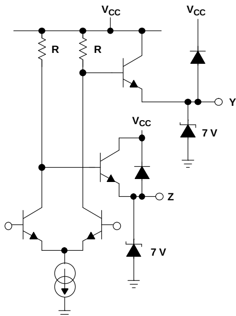
OUTPUT LVP18/19
