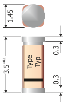
Dimensions - Maße [mm]
