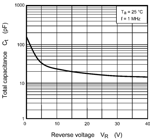
Fig. 9.3 C_t - V_R
