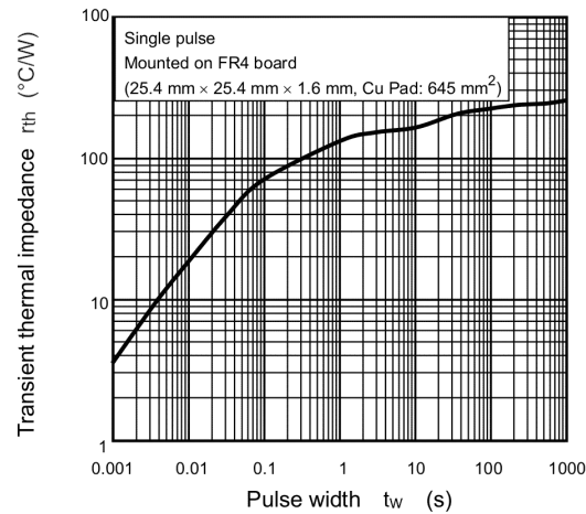
Fig. 7.12 r_{th} - t_w
