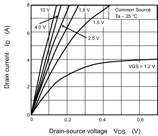
Fig. 7.1 I_D - V_{DS}
