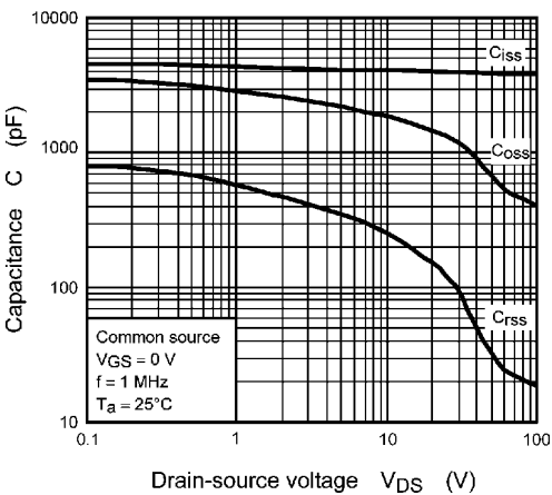
Fig. 8.11 Capacitance - V_{DS}
