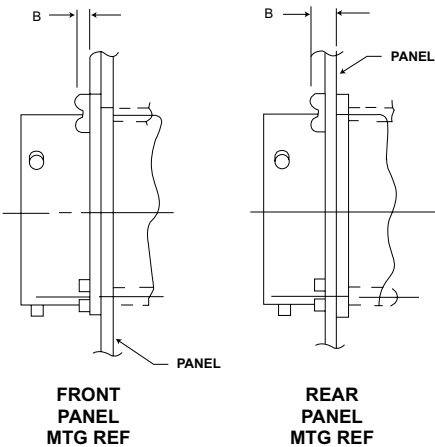
Thru-Bulkhead Receptacle
