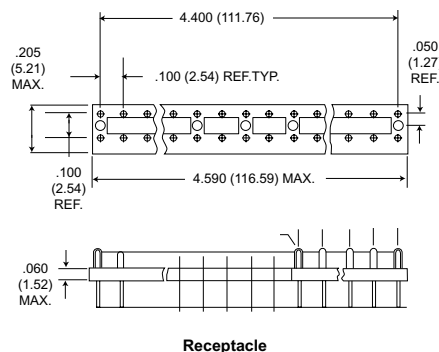
Receptacle
