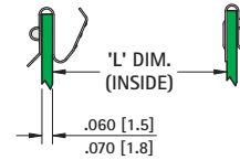
Fig. 1 Spring-Button
