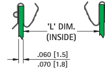
Fig. 2 Spring-Spring
