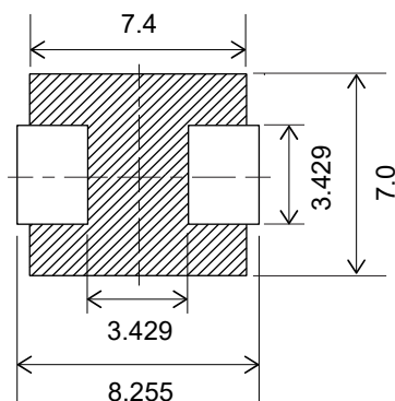
PCC-M0630M-LP type (ETQP3M□□□KVN)
