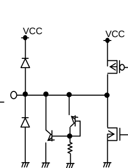
19pin&lt;PERST#&gt;
