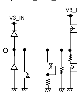
3,4pin&lt;V3_1,V3_2&gt;
