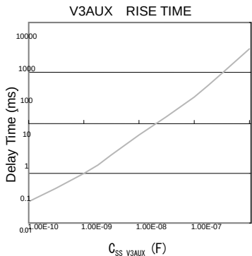
Fig.12 V3AUX RISE TIME
