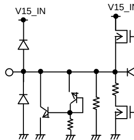
8,9pin&lt;V15_1,V15_2&gt;
