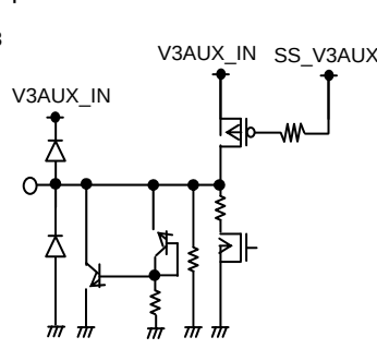
5pin&lt;V3AUX&gt;
