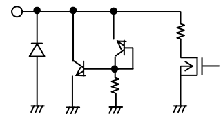
15pin&lt;OC&gt;
