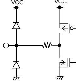
14pin&lt;OC_DELAY&gt;
