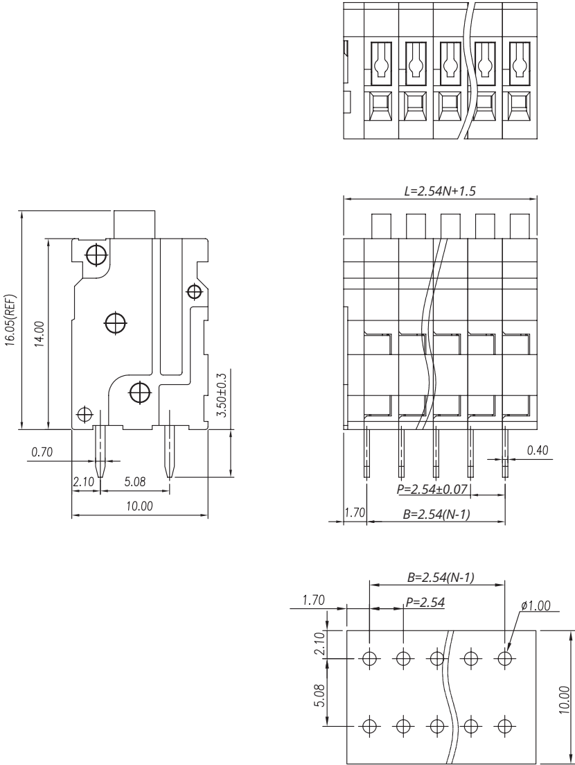
P.C.B. LAYOUT
