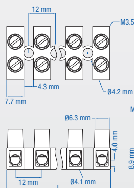
HE6 DIMENSIONS
