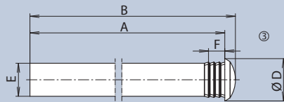
Montagebohrung C Mounting hole C
