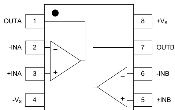
SOIC-8/MSOP-8
