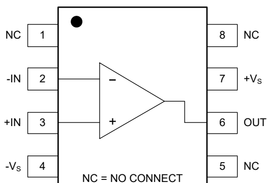
SOIC-8/MSOP-8
