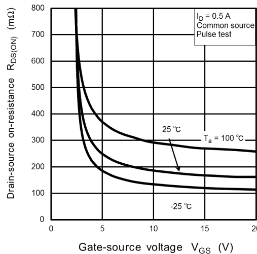
Fig. 8.4 R_{DS(ON)} - V_{GS}
