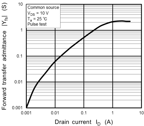
Fig. 8.9 |Y_{fs}| - I_D
