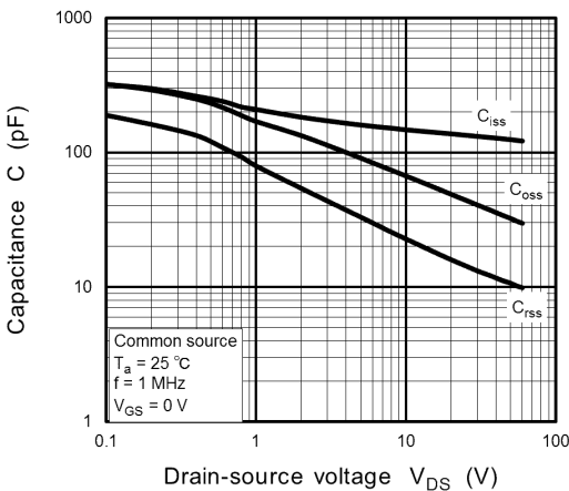
Fig. 8.11 C - V_{DS}
