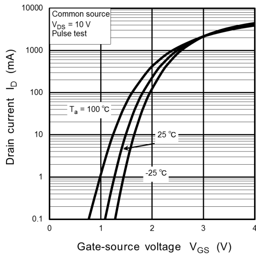
Fig. 8.3 I_D - V_{GS}
