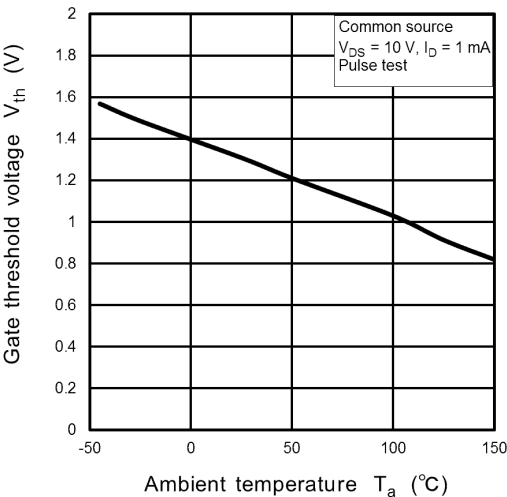
Fig. 8.8 V_{th} - T_a
