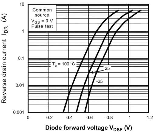
Fig. 8.10 I_{DR} - V_{DSF}
