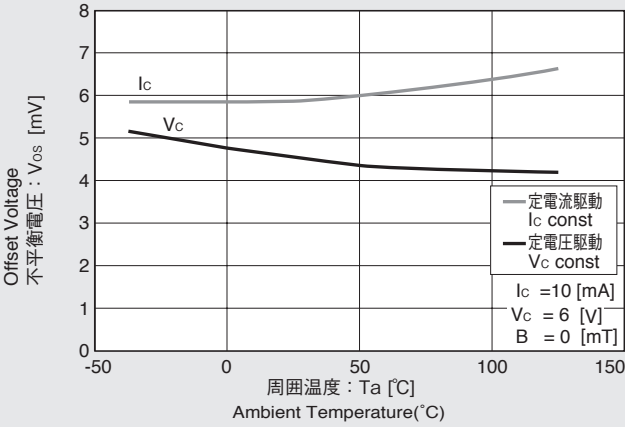
V os (V u )-T (参考)
