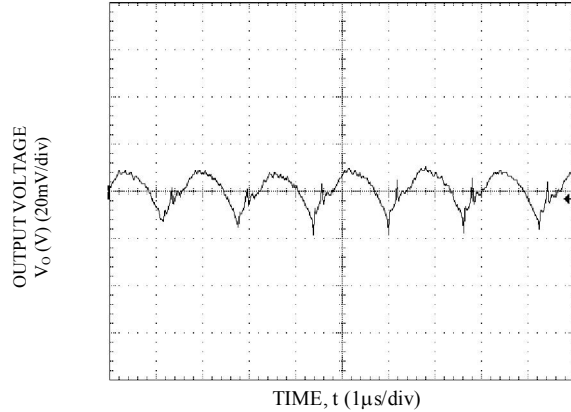
Vo=1.2V, Io = Io,max, Vin=12V
