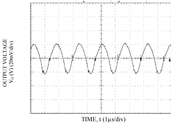
Vo=3.3V, Io = Io,max, Vin=12V
