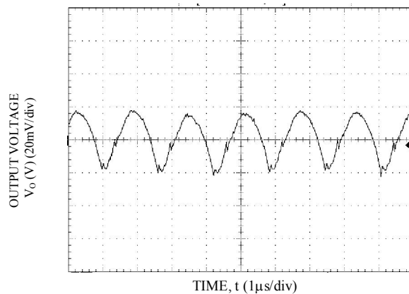
Vo=2.5V, Io = Io,max, Vin=12V
