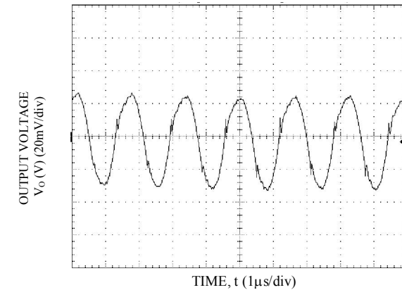
Vo=5.0V, Io = Io,max, Vin=12V
