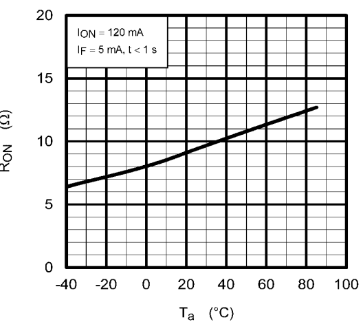
Fig. 12.1.5 R_{ON} - T_a
