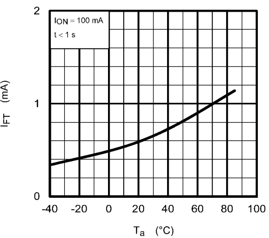
Fig. 12.1.6 I_{FT} - T_a
