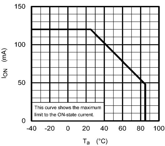
Fig. 12.1.2 I_{ON} - T_a
