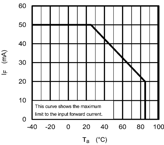
Fig. 12.1.1 I_F - T_a
