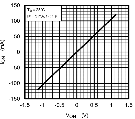
Fig. 12.1.4 I_{ON} - V_{ON}
