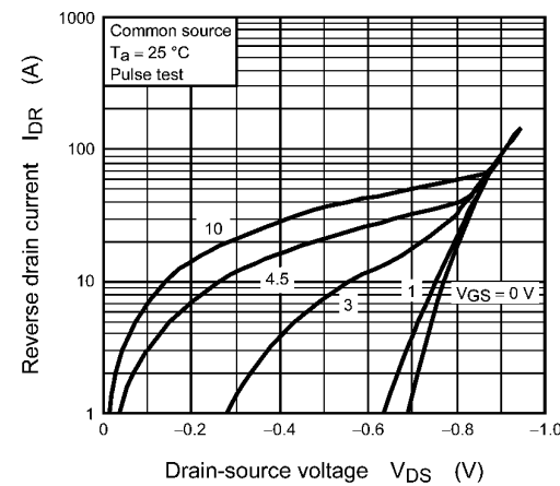
Fig. 8.6 I_{DR} - V_{DS}
