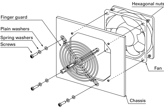
Axial fan
