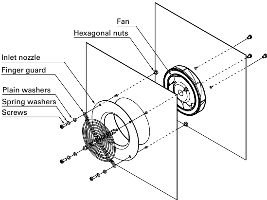
Centrifugal fan
