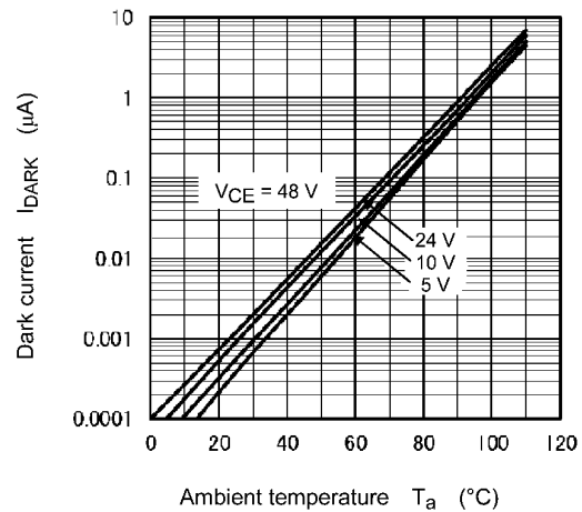
Fig. 11.10 I_{\text{DARK}} - T_a
