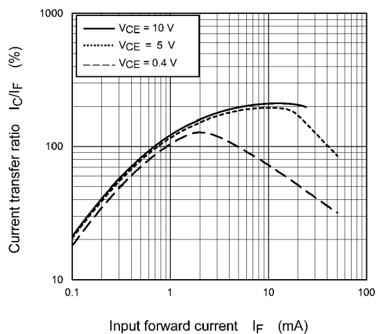
Fig. 11.11 I_C/I_F - I_F
