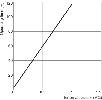
H3FA-A/-SA/-AU/-SAU
