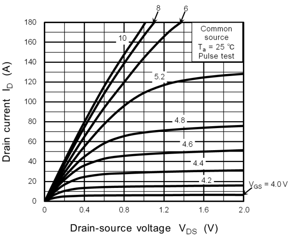
Fig. 8.2 I_D - V_{DS}
