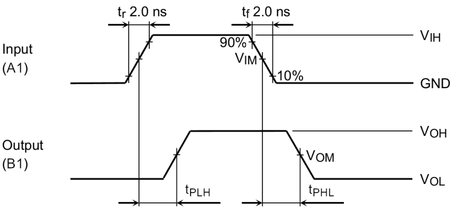
Fig. 13.1 t_{PLH} , t_{PHL}
