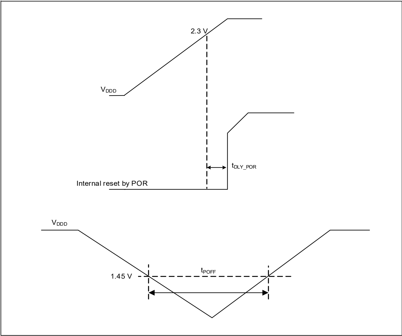
Figure 25 POR specifications
