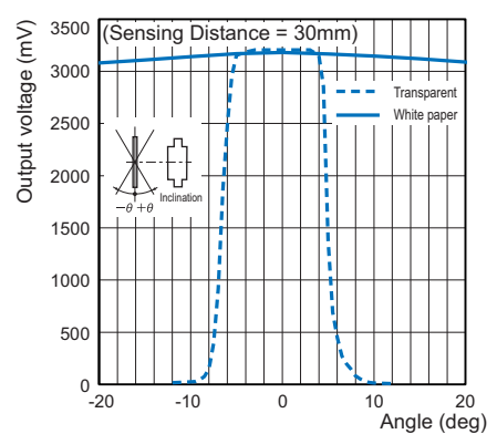
B5W-LB2101
