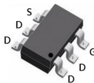
SOT-23-6
