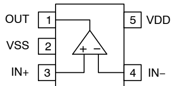
SOT23-5 / TSOP-5
