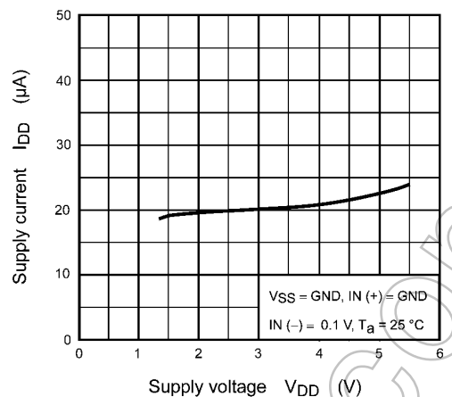
Fig. 10.9 I_{DD} - V_{DD}
