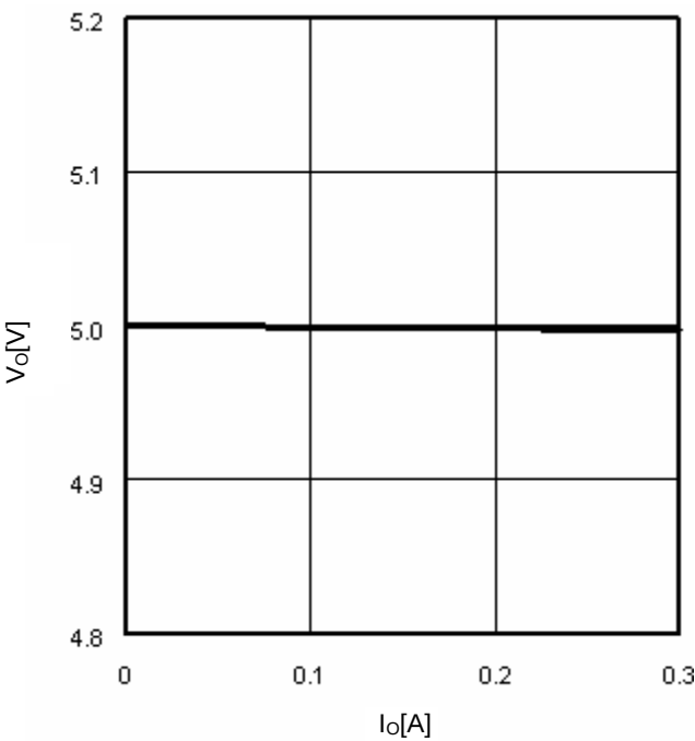
Fig.13 Io-V O
