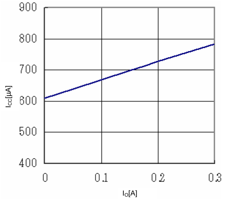
Fig.20 I_o - I_{cc}
