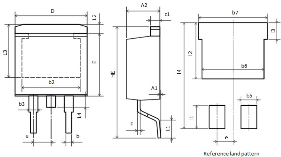
TO-263AB (TO-263AB-3LSHYAD)
