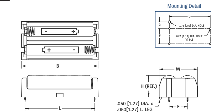
DWG. 4
