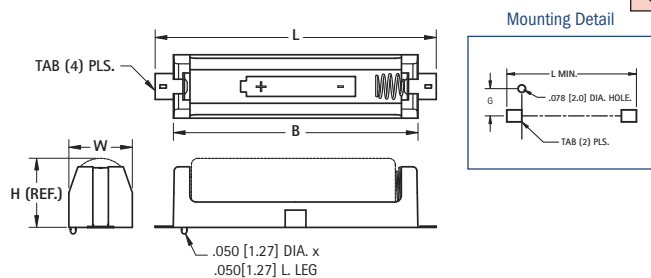
DWG. 1
