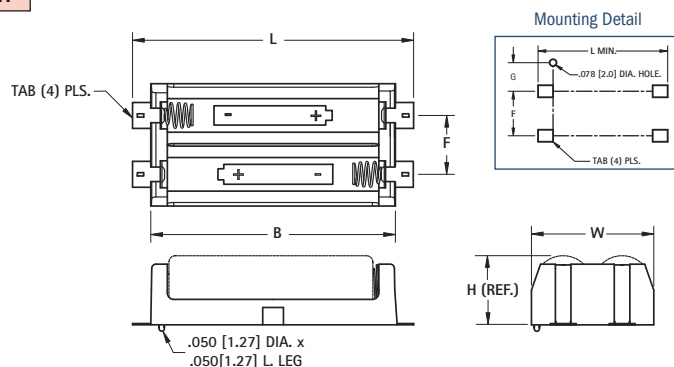
DWG. 2
