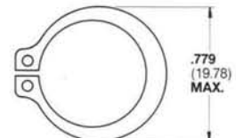
SIZE 24 990-0014-063
