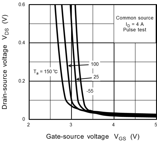
Fig. 8.5 V_{DS} - V_{GS}
