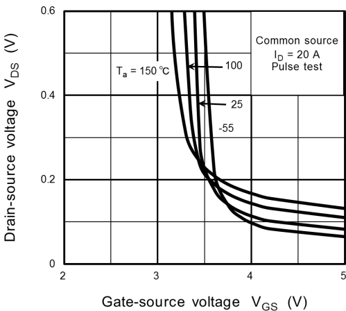
Fig. 8.3 V_{DS} - V_{GS}
