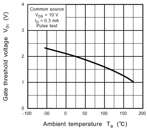
Fig. 8.12 V_{th} - T_a
