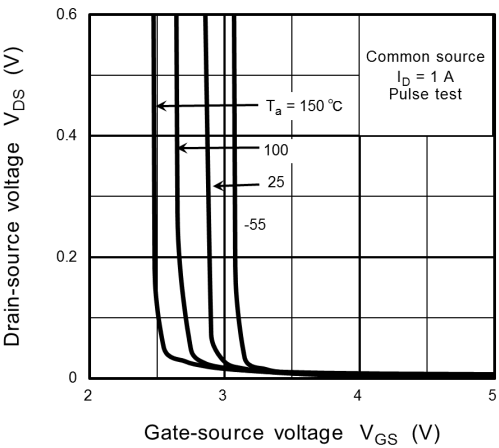
Fig. 8.6 V_{DS} - V_{GS}
