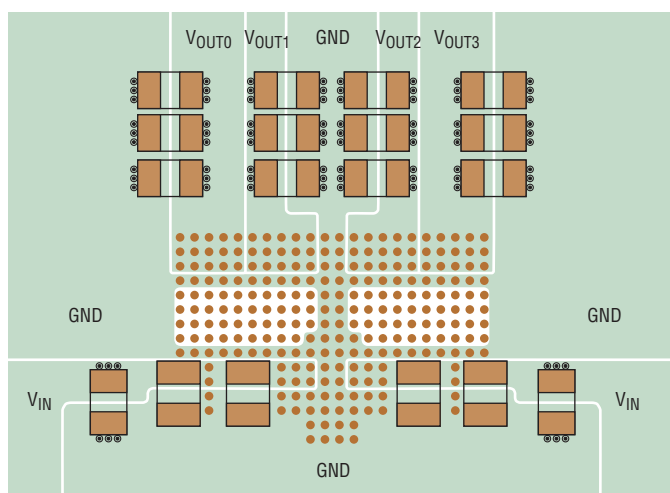
(b) LTM4681 BOTTOM LAYER
