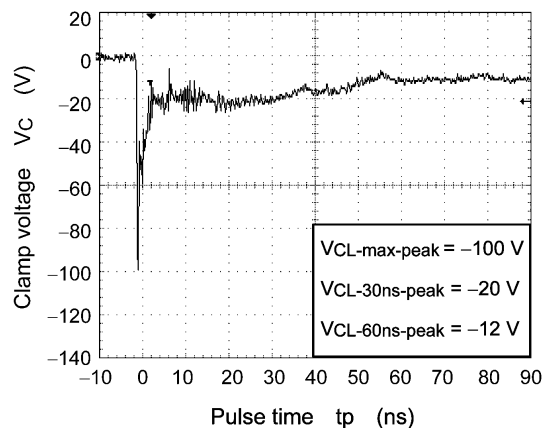
Fig. 6.1.2 -8 kV
