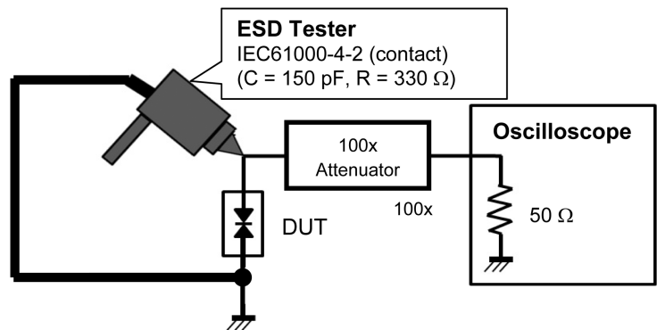
Fig. 6.1.5 IEC61000-4-2 (Contact)
