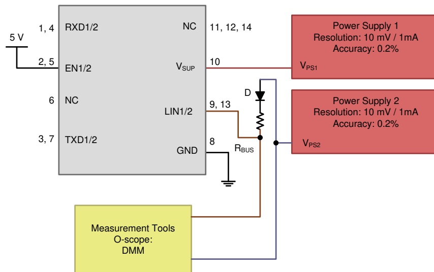
Figure 7-5. V_{SUP\_NON\_OP} Parameters 11
