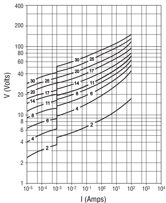
Model Size 0805 - (ZV 2 M 0805 xxx ~ ZV 30 K 0805 xxx)
