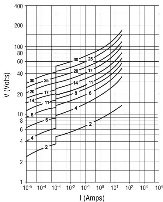
Model Size 0603 - (ZV 2 M 0603 300 ~ ZV 30 K 0603 300)
