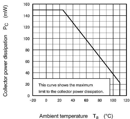
Fig. 11.2 P_C - T_a
