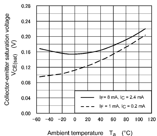
Fig. 11.12 V_{CE(\text{sat})} - T_a
