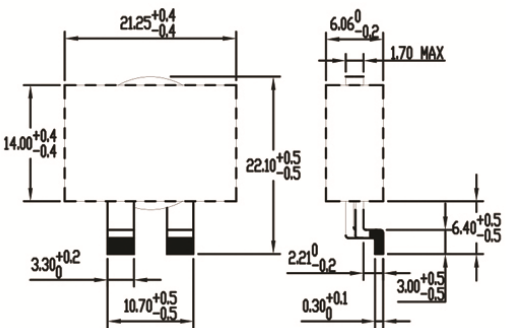
PQ3213-0R9-70-G | 0.9 μH
