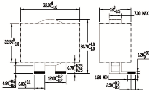
PQ3218-3R3-70-T | 3.3 μH
