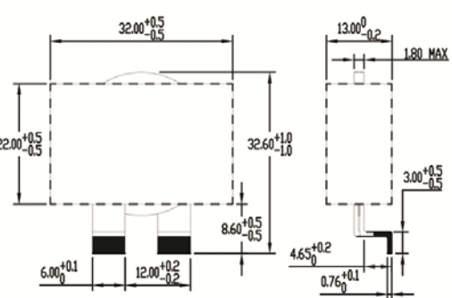
PQ3218-6R0-50-T - 6.0 μH
