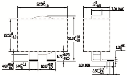
PQ3218-6R0-50-T - 6.0 μH
