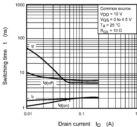
Fig. 7.11 t - I_D
