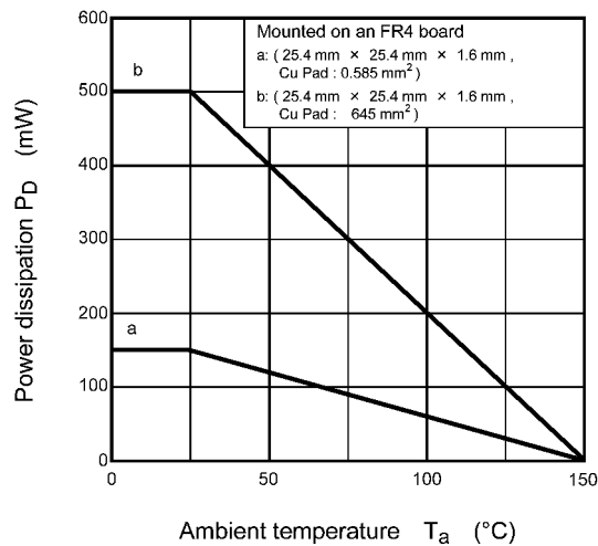
Fig. 7.13 P_D - T_a
