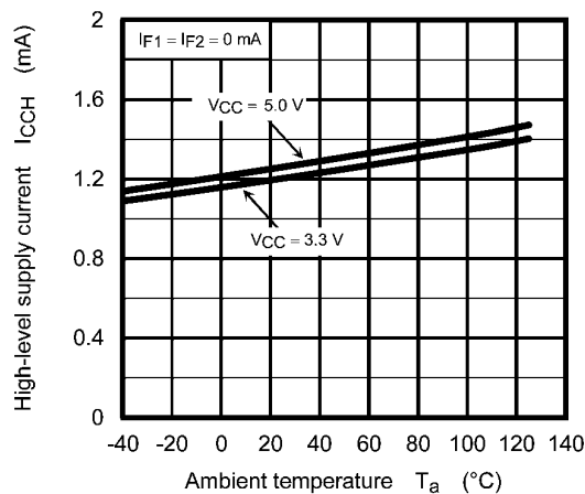
Fig. 12.2.8 I_{CCH} - T_a
