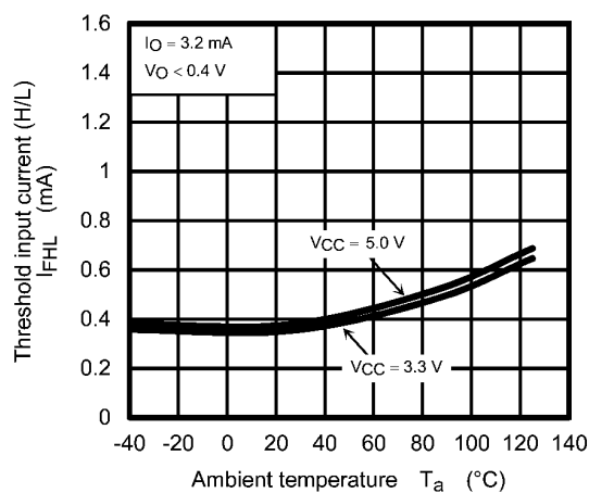
Fig. 12.2.9 I_{FHL} - T_a
