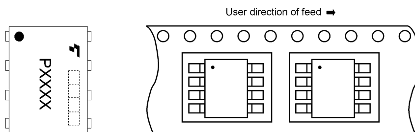
Fig. 17.3.1.1 Device Orientation
