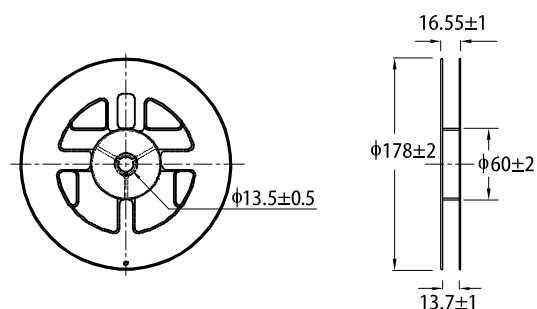
REEL DIMENSION (units : mm)
