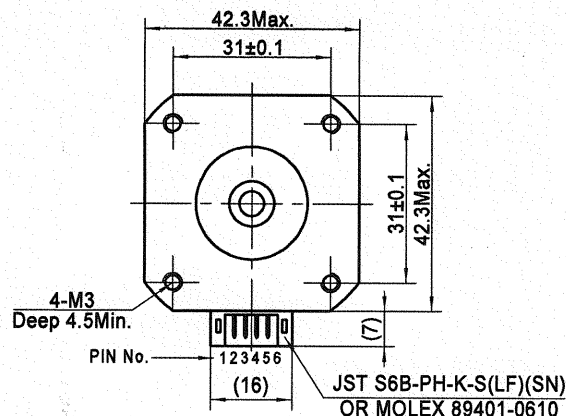
接线图
